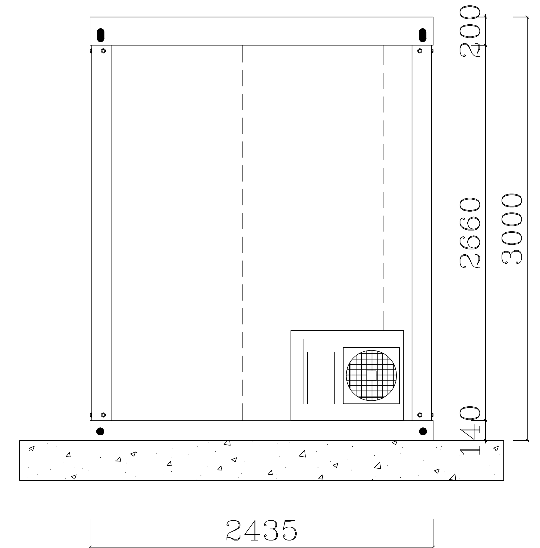
PROSPETTO 1
