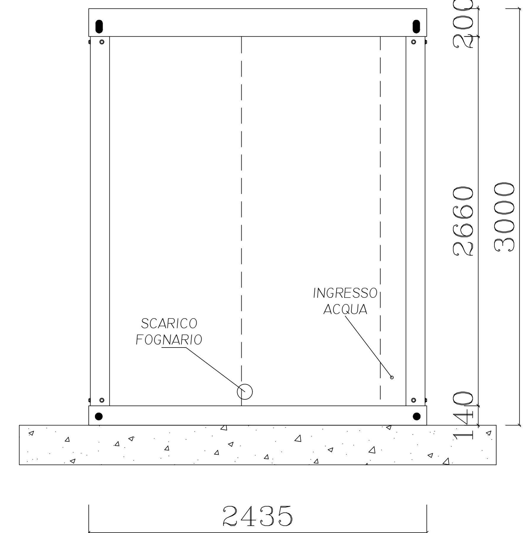
PROSPETTO 3
